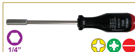
IMPUGNATURA PORTA INSERTI CON MAGNETE + SERBATOIO CON 6 INSERTI: - PH 1, PH 2 - PZ 1, PZ 2 - TAGLIO: 0.8 X 4.0 - 1.0 X 5.5
